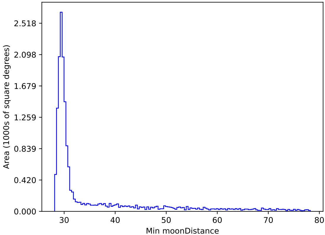
no_high_blob_v3.3_10yrs WFD y band: Min moonDistance
