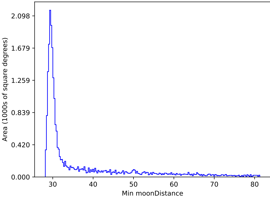
no_high_blob_v3.3_10yrs All sky y band: Min moonDistance
