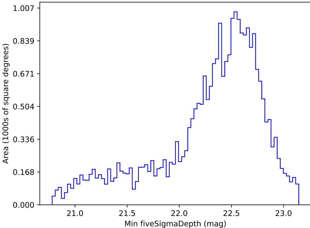
no_high_blob_v3.3_10yrs Yr 1 z band: Min fiveSigmaDepth
