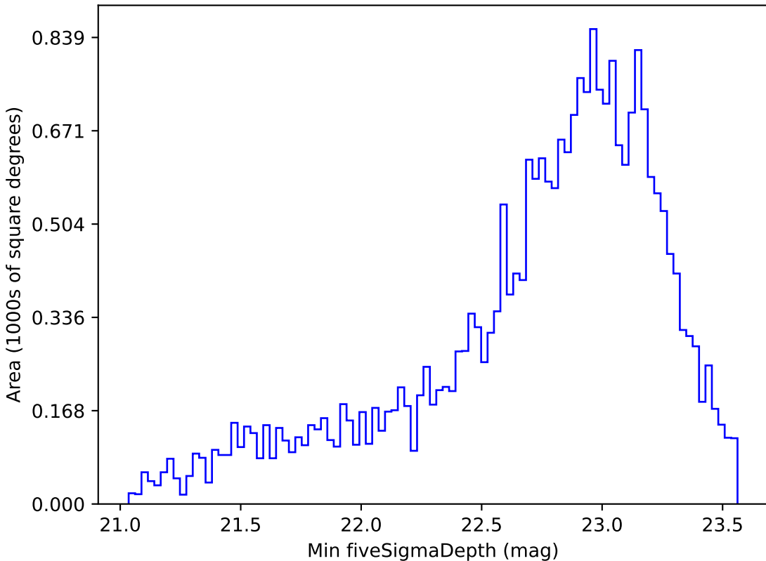
no_high_blob_v3.3_10yrs Yr 1 i band: Min fiveSigmaDepth
