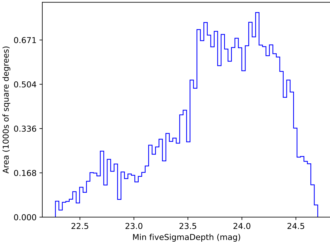
no_high_blob_v3.3_10yrs Yr 1 g band: Min fiveSigmaDepth
