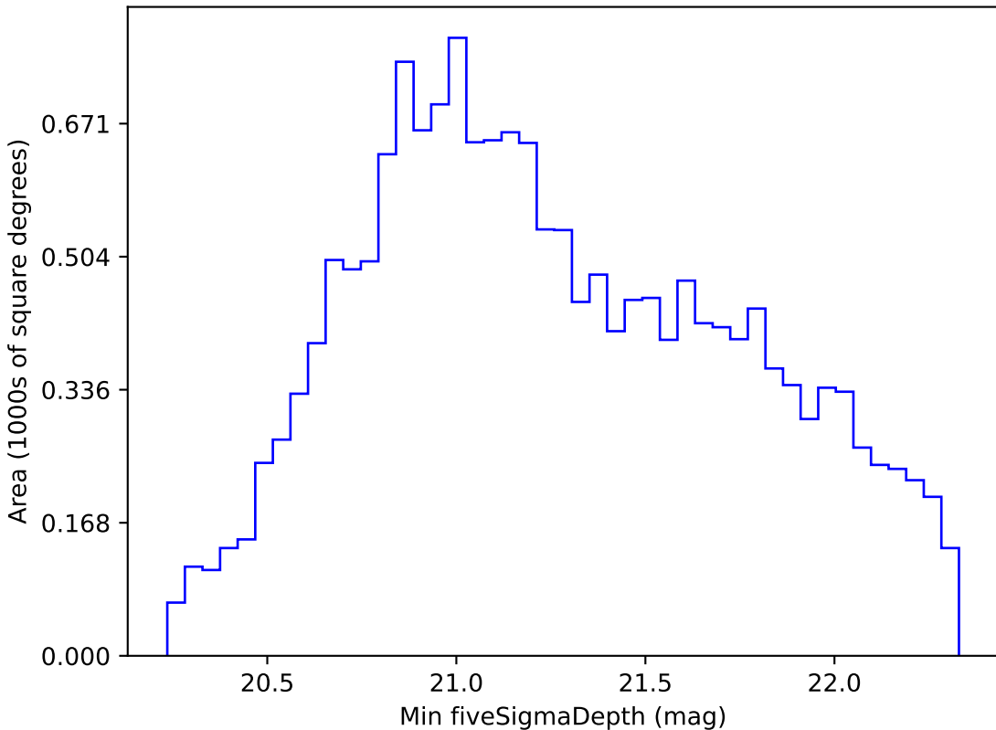
no_high_blob_v3.3_10yrs WFD z band: Min fiveSigmaDepth
