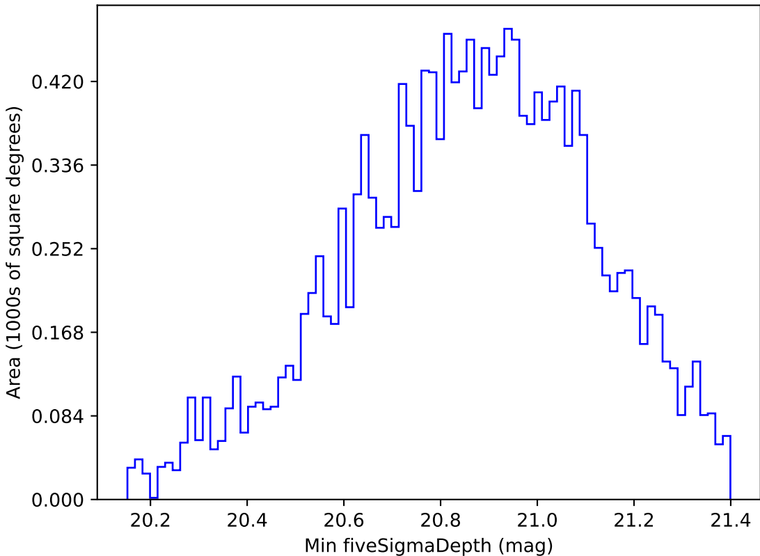
no_high_blob_v3.3_10yrs WFD y band: Min fiveSigmaDepth
