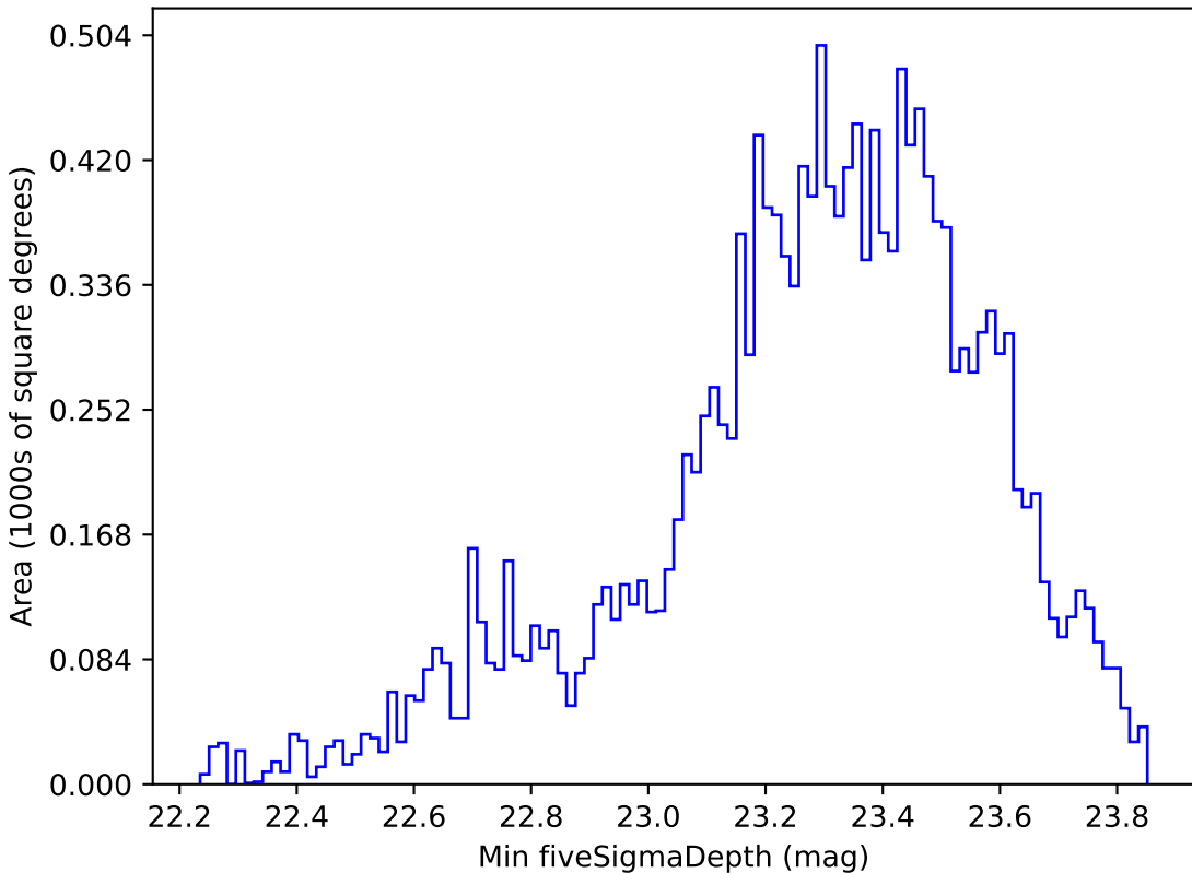
no_high_blob_v3.3_10yrs WFD g band: Min fiveSigmaDepth
