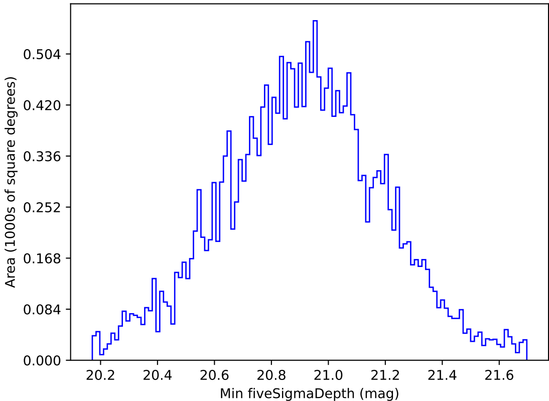
no_high_blob_v3.3_10yrs All sky y band: Min fiveSigmaDepth
