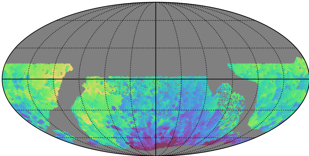
no_high_blob_v3.3_10yrs WFD y band: Min HA
