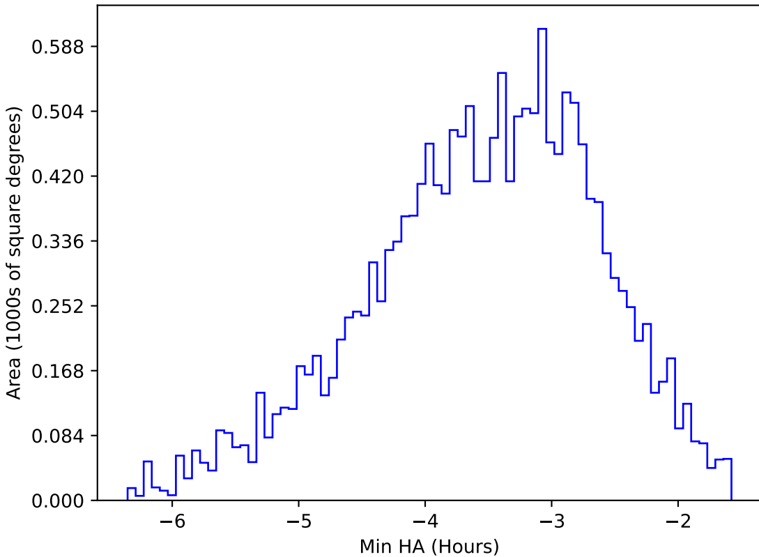
no_high_blob_v3.3_10yrs WFD y band: Min HA
