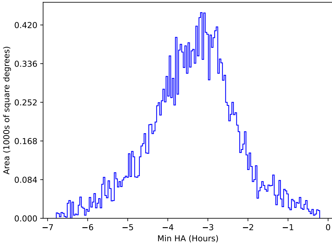
no_high_blob_v3.3_10yrs All sky y band: Min HA
