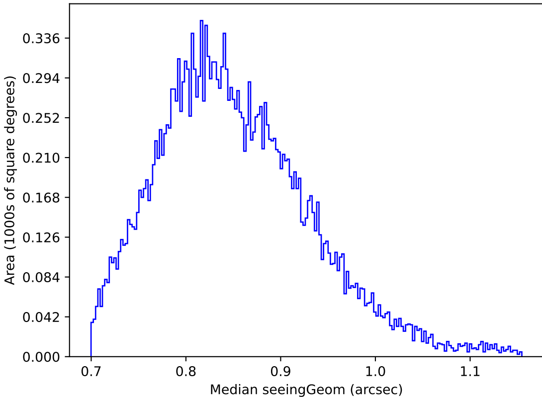
no_high_blob_v3.3_10yrs Yr 1 y band: Median seeingGeom
