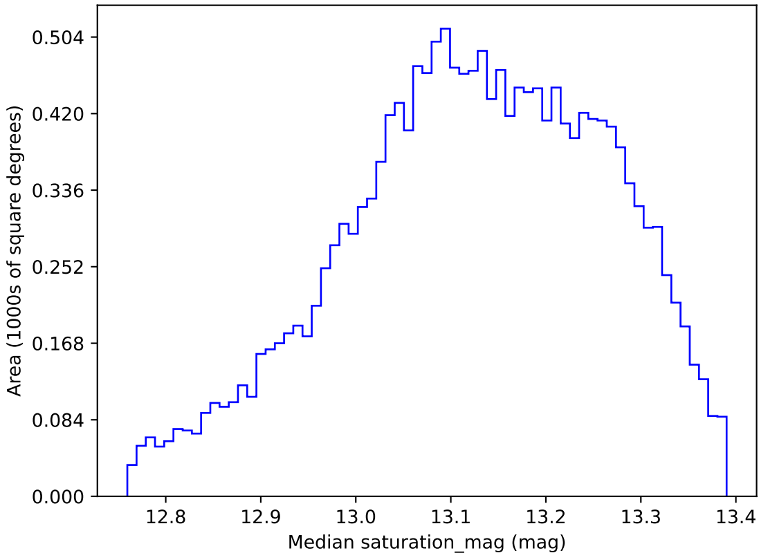
no_high_blob_v3.3_10yrs WFD y band: Median saturation_mag
