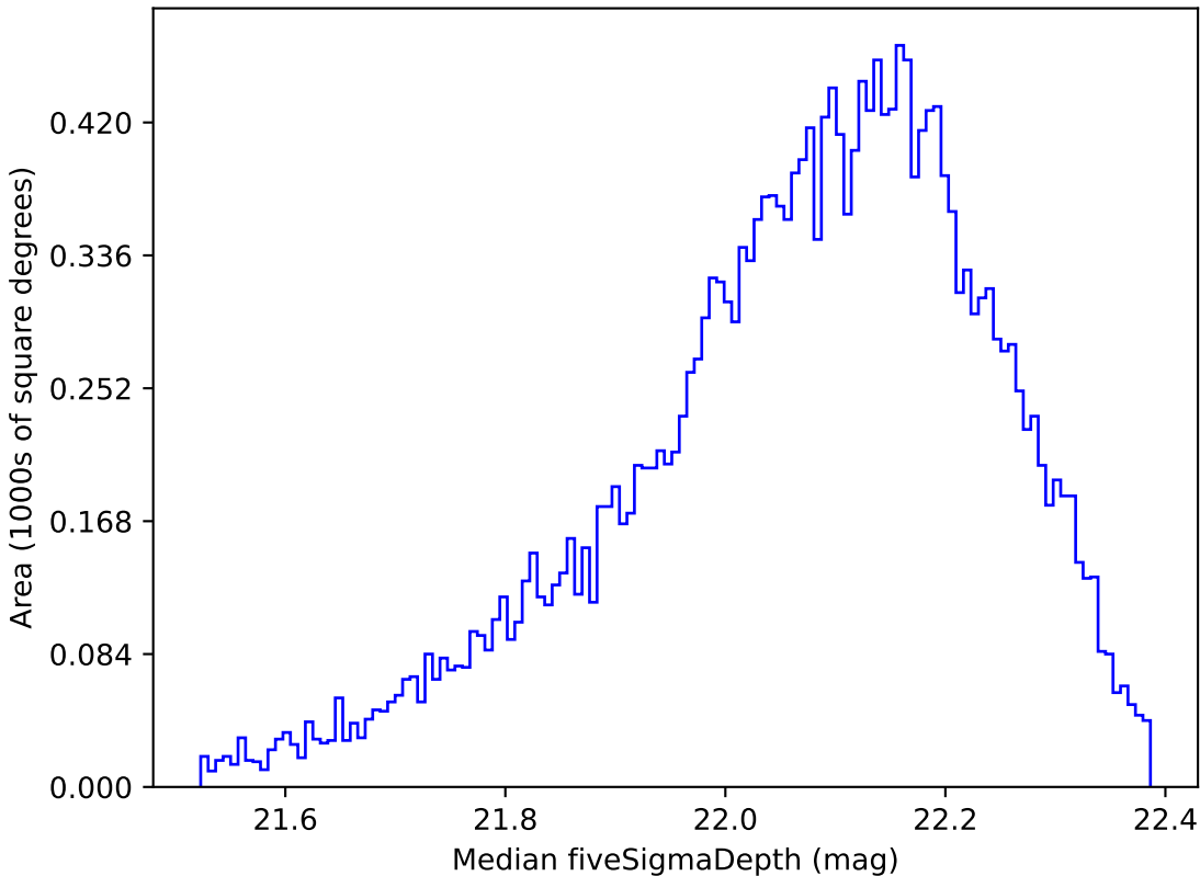
no_high_blob_v3.3_10yrs Yr 1 y band: Median fiveSigmaDepth
