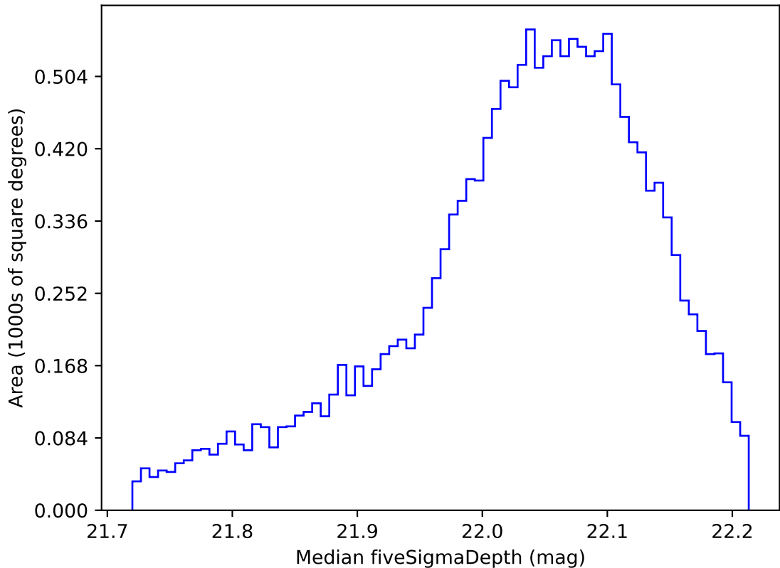
no_high_blob_v3.3_10yrs WFD y band: Median fiveSigmaDepth
