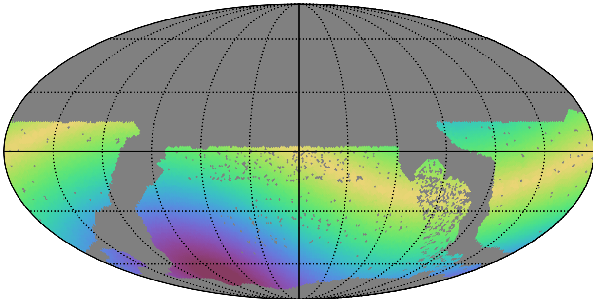
no_high_blob_v3.3_10yrs WFD y band: Max solarElong
