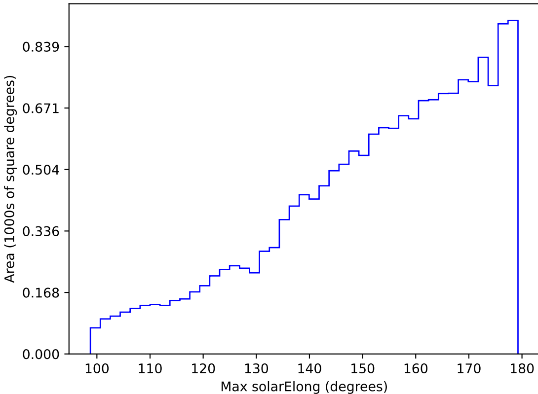
no_high_blob_v3.3_10yrs WFD y band: Max solarElong
