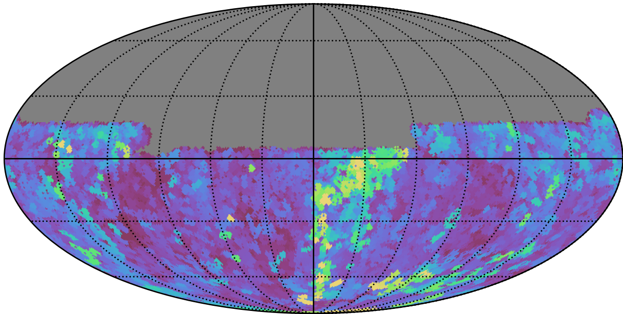
no_high_blob_v3.3_10yrs Yr 1 y band: Max seeingGeom
