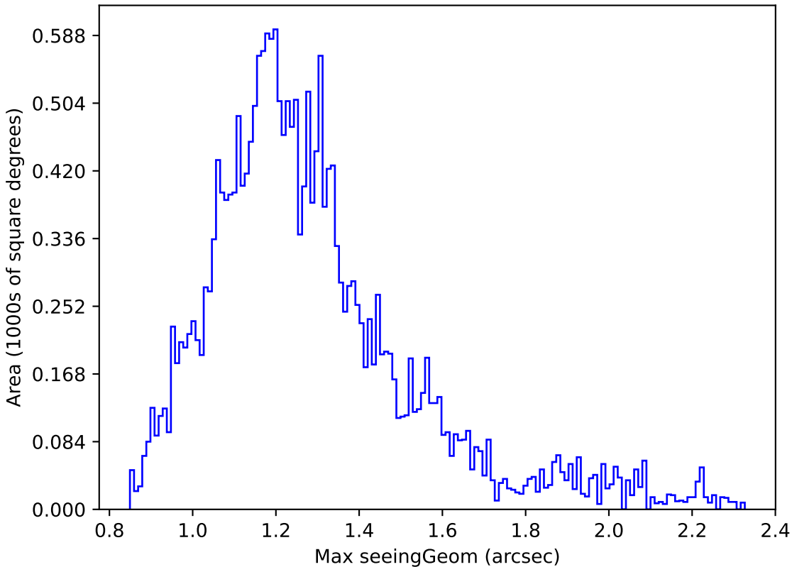
no_high_blob_v3.3_10yrs Yr 1 y band: Max seeingGeom
