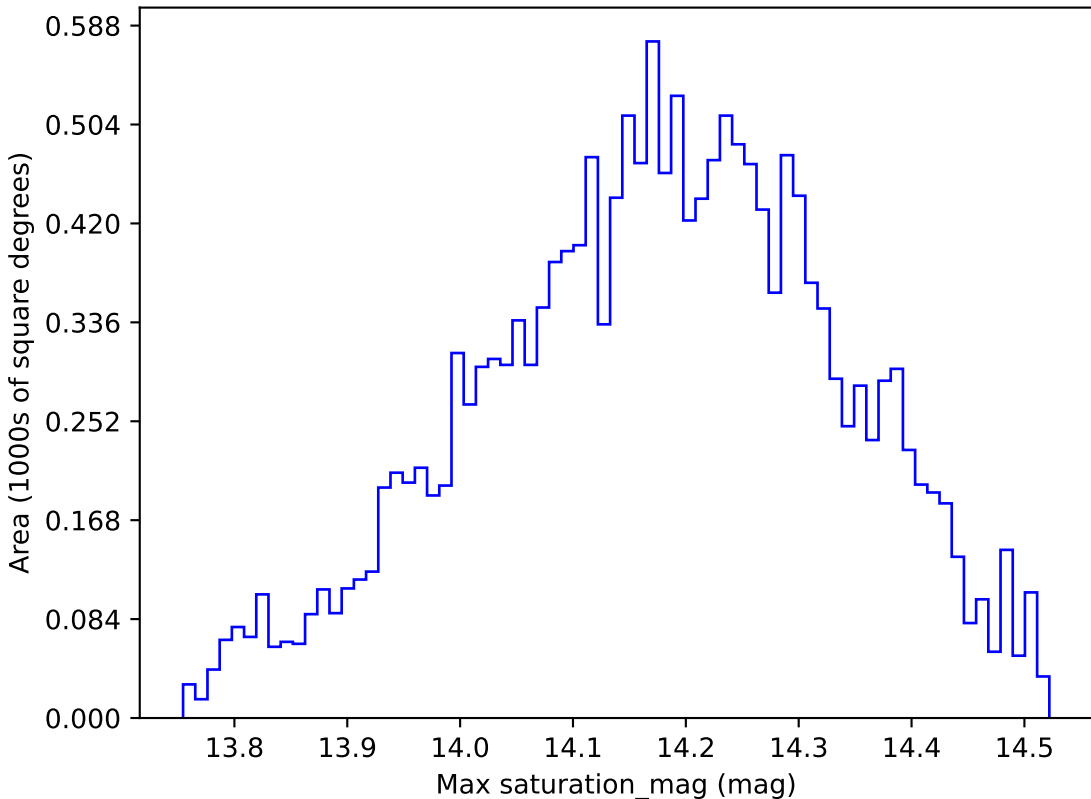
no_high_blob_v3.3_10yrs WFD y band: Max saturation_mag
