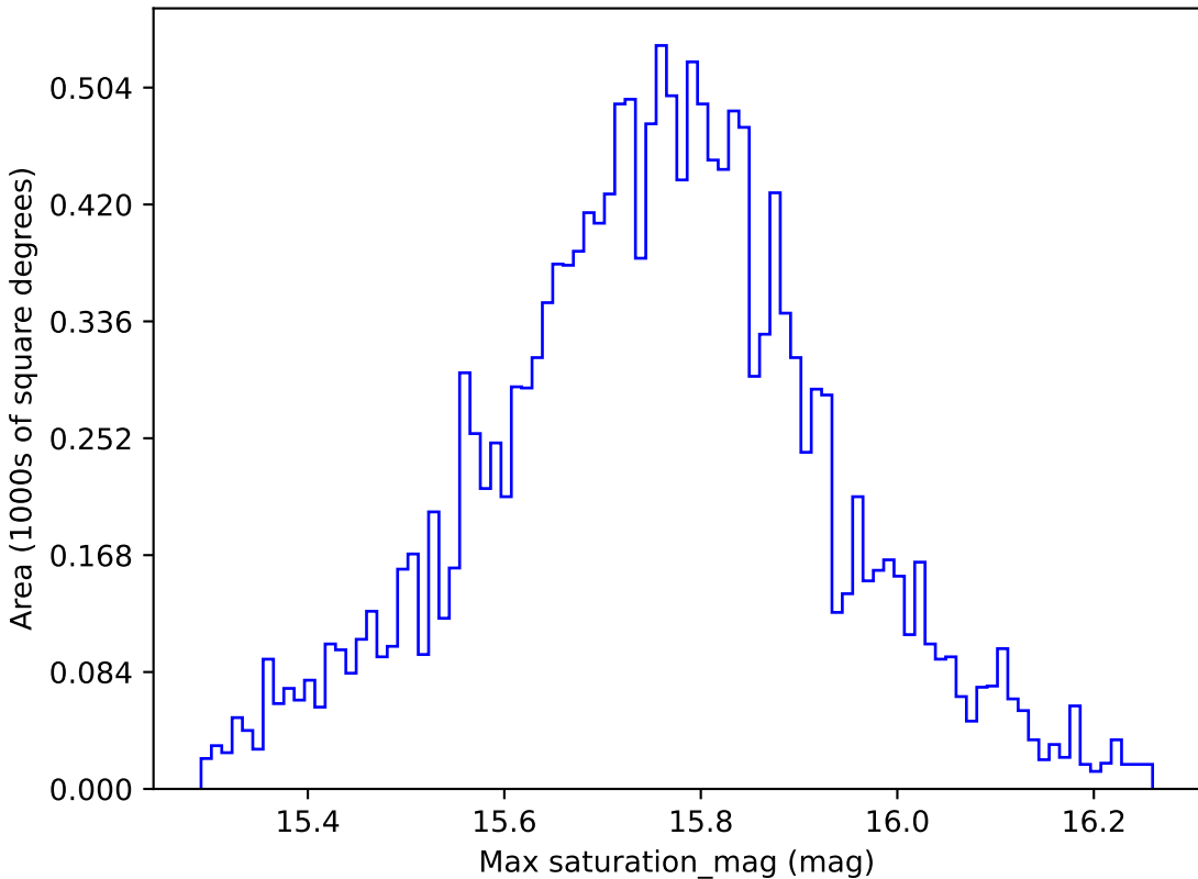
no_high_blob_v3.3_10yrs WFD g band: Max saturation_mag
