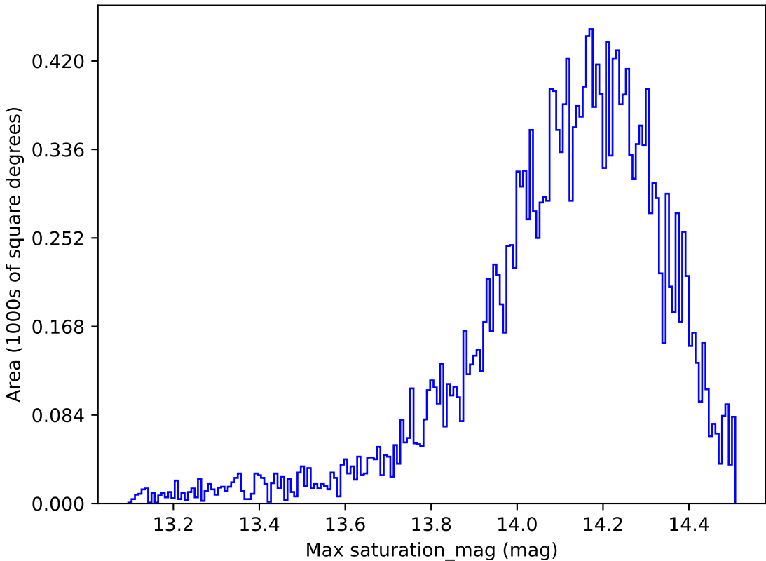
no_high_blob_v3.3_10yrs All sky y band: Max saturation_mag
