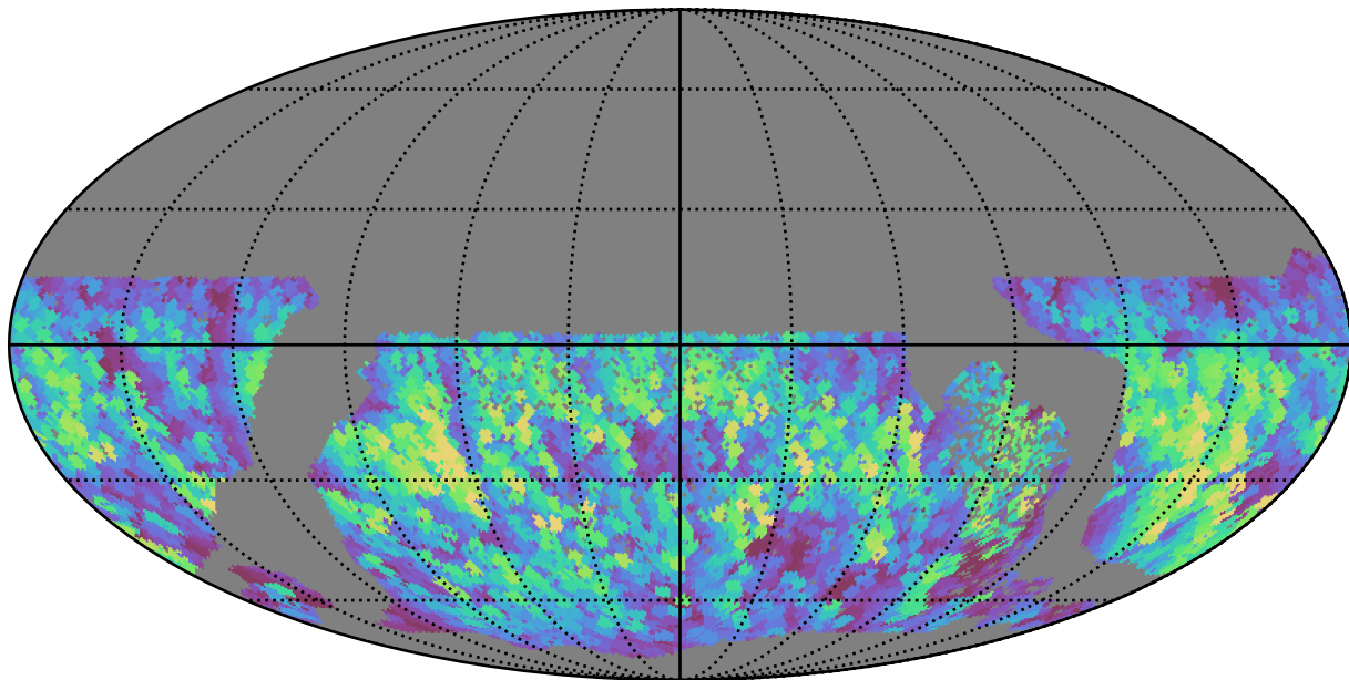
no_high_blob_v3.3_10yrs WFD y band: Max normairmass
