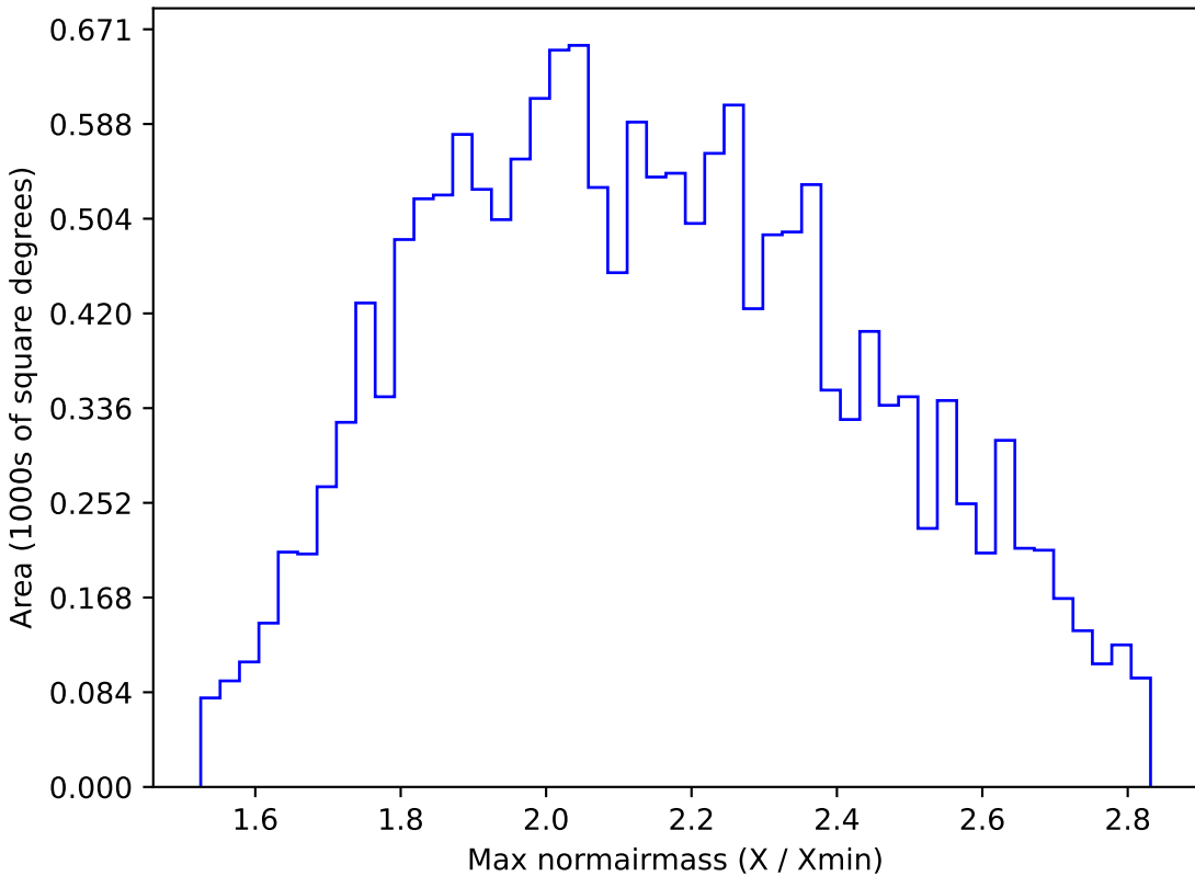
no_high_blob_v3.3_10yrs WFD y band: Max normairmass
