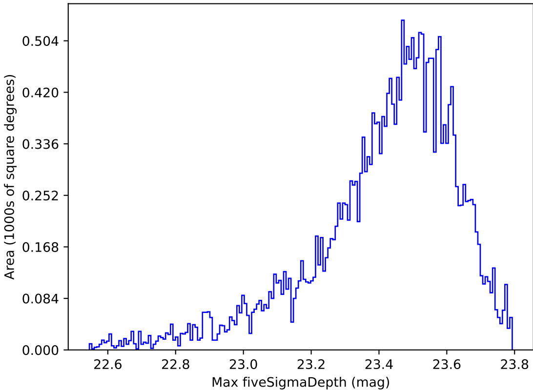
no_high_blob_v3.3_10yrs Yr 1 z band: Max fiveSigmaDepth
