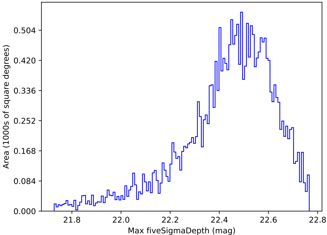
no_high_blob_v3.3_10yrs Yr 1 y band: Max fiveSigmaDepth
