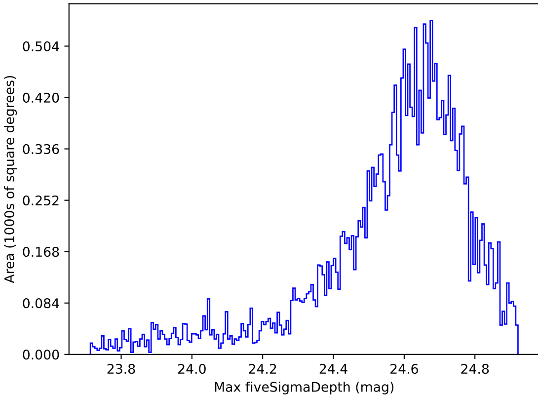
no_high_blob_v3.3_10yrs Yr 1 r band: Max fiveSigmaDepth
