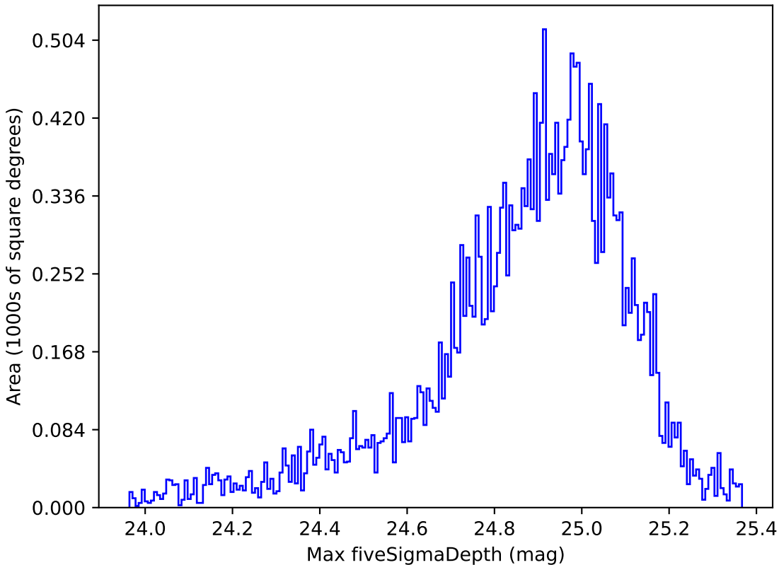
no_high_blob_v3.3_10yrs Yr 1 g band: Max fiveSigmaDepth
