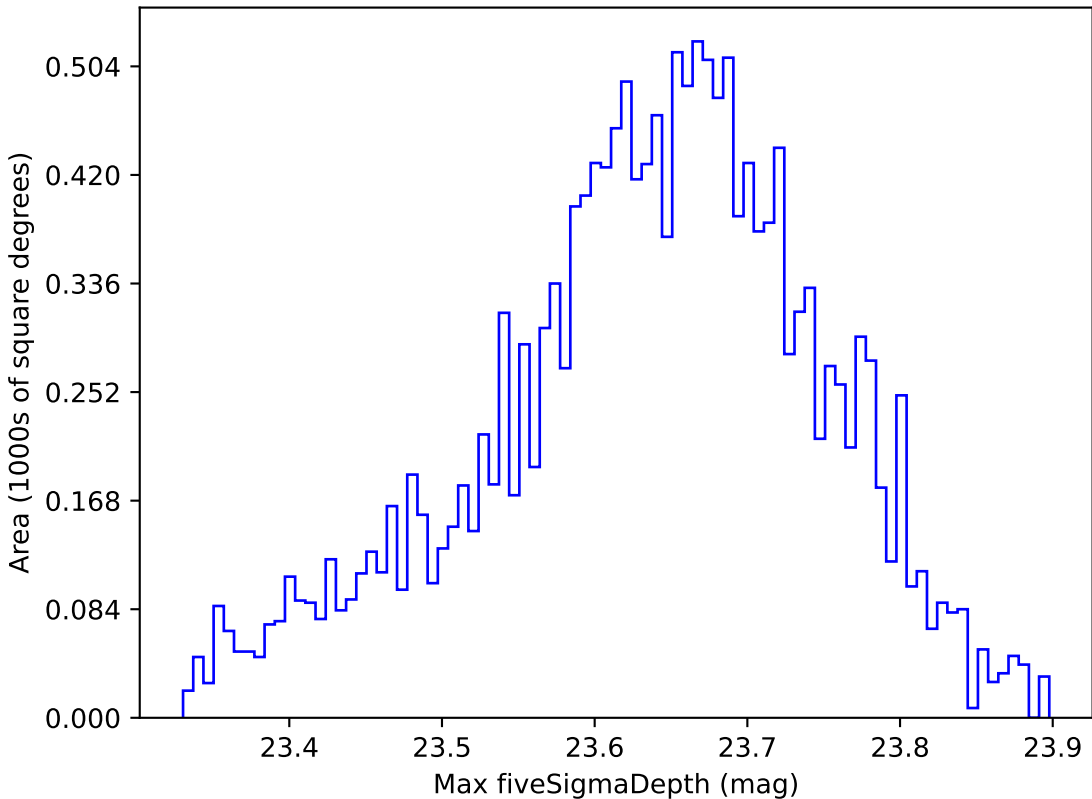
no_high_blob_v3.3_10yrs WFD z band: Max fiveSigmaDepth
