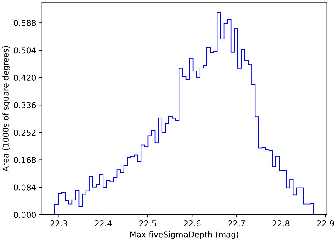
no_high_blob_v3.3_10yrs WFD y band: Max fiveSigmaDepth
