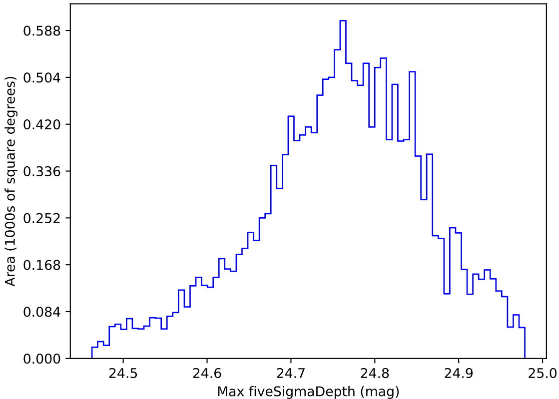
no_high_blob_v3.3_10yrs WFD r band: Max fiveSigmaDepth
