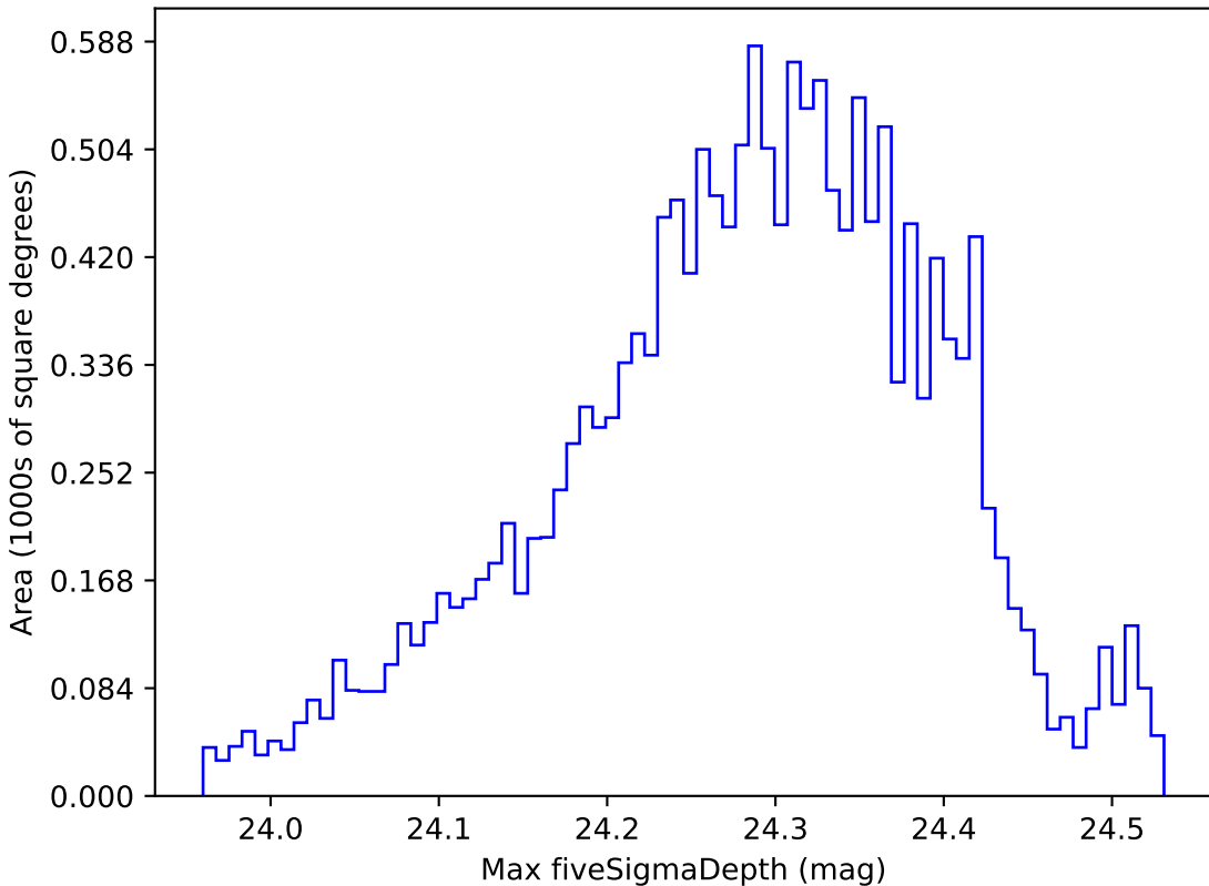
no_high_blob_v3.3_10yrs WFD i band: Max fiveSigmaDepth
