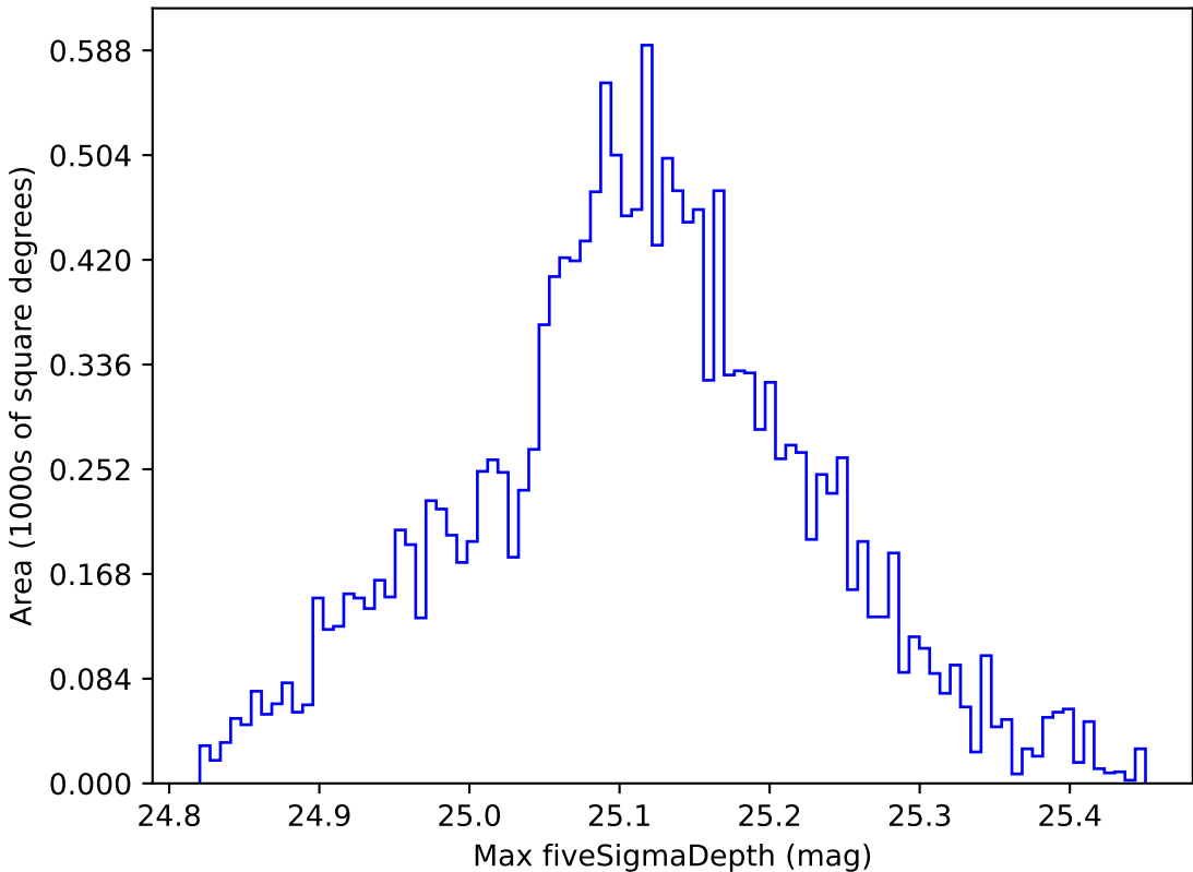
no_high_blob_v3.3_10yrs WFD g band: Max fiveSigmaDepth
