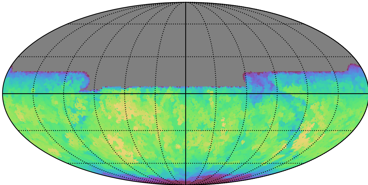
no_high_blob_v3.3_10yrs All sky y band: Max fiveSigmaDepth
