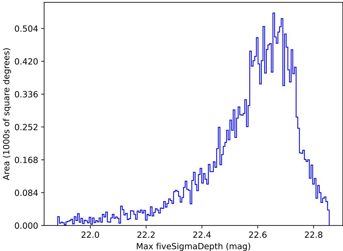
no_high_blob_v3.3_10yrs All sky y band: Max fiveSigmaDepth
