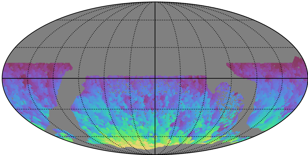
no_high_blob_v3.3_10yrs WFD y band: Max HA
