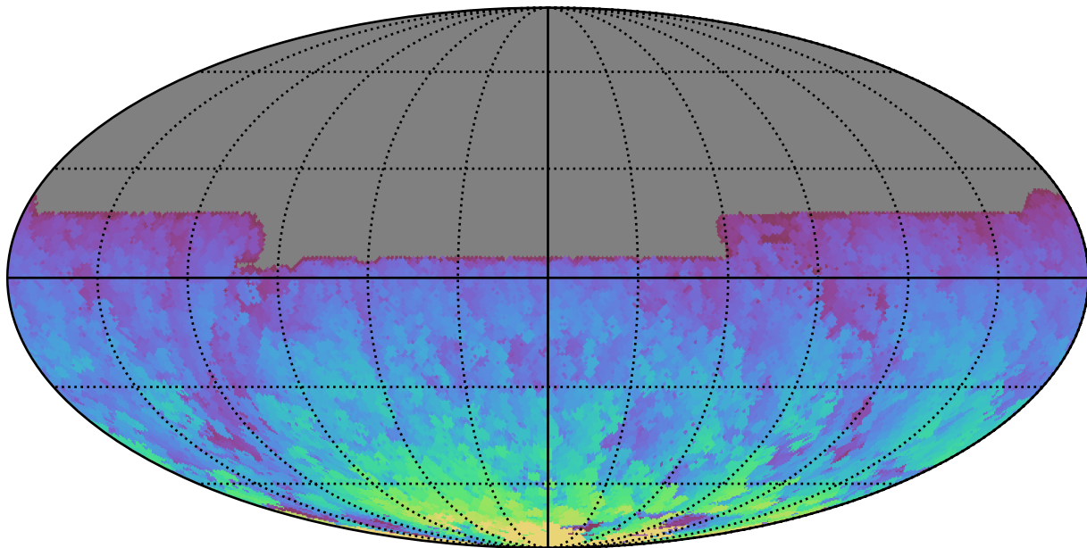
no_high_blob_v3.3_10yrs All sky y band: Max HA
