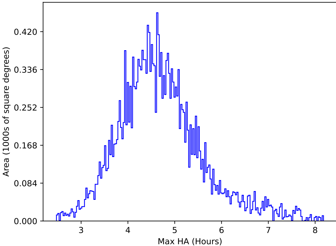
no_high_blob_v3.3_10yrs All sky y band: Max HA
