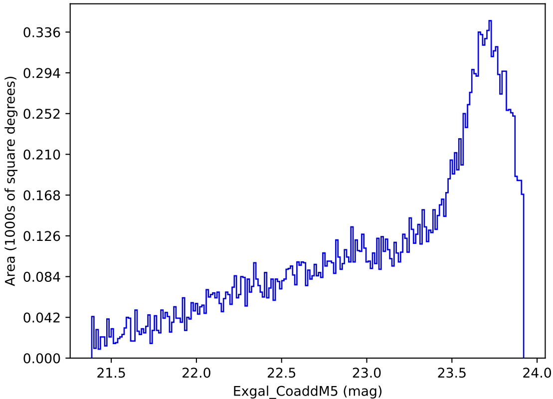
no_high_blob_v3.3_10yrs Yr 3-4 y band: Exgal_CoaddM5
