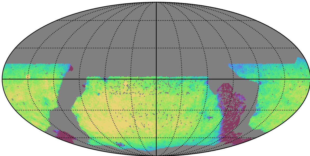
no_high_blob_v3.3_10yrs WFD y band: Exgal_CoaddM5
