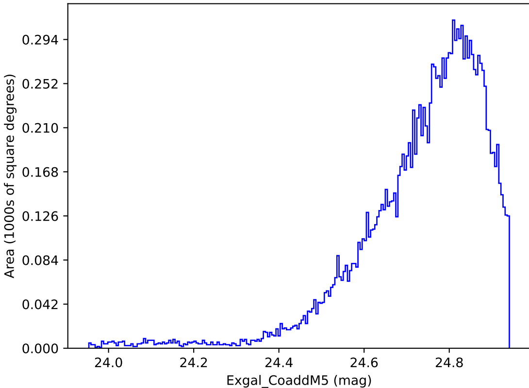
no_high_blob_v3.3_10yrs WFD y band: Exgal_CoaddM5
