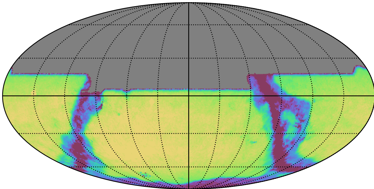
no_high_blob_v3.3_10yrs All sky y band: Exgal_CoaddM5
