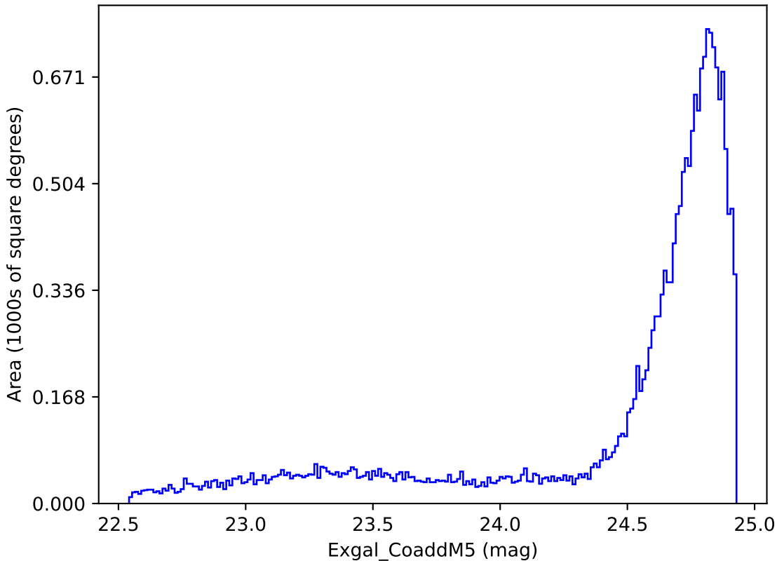
no_high_blob_v3.3_10yrs All sky y band: Exgal_CoaddM5
