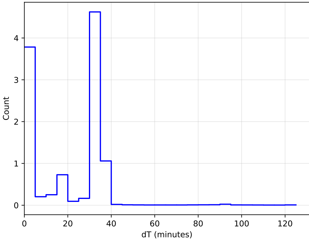
1e6 no_high_blob_v3.3_10yrs WFD: DeltaT Histogram
