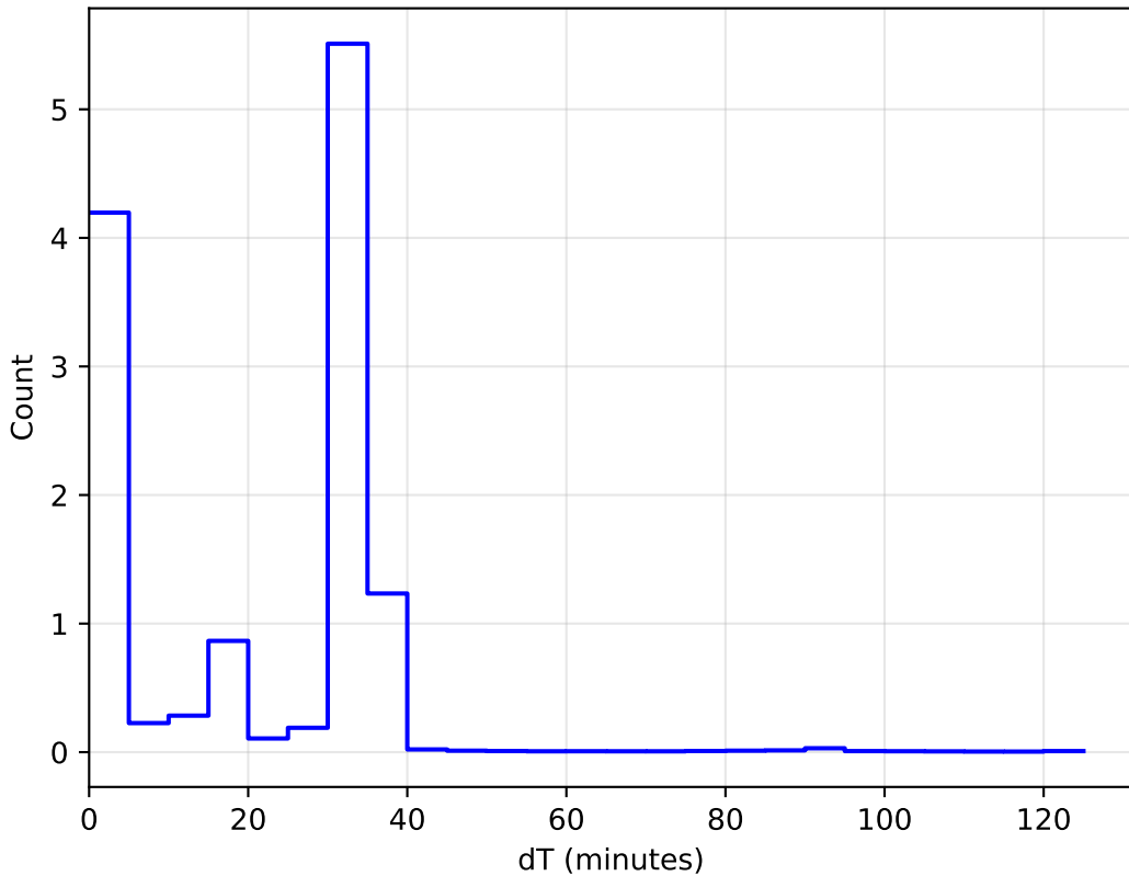
1e6 no_high_blob_v3.3_10yrs All sky: DeltaT Histogram
