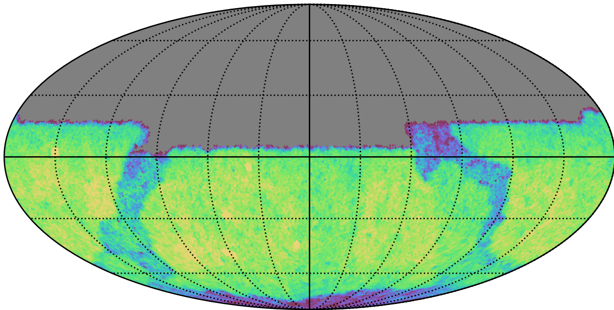
no_high_blob_v3.3_10yrs Yr 1 y band: CoaddM5
