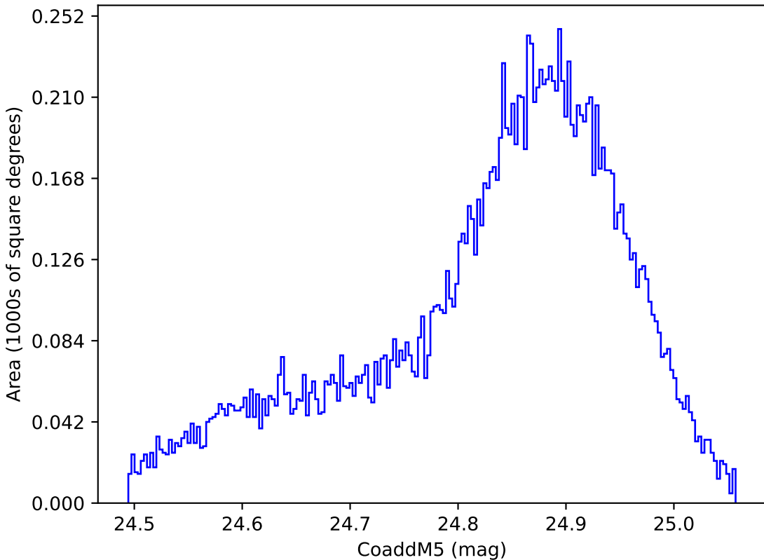
no_high_blob_v3.3_10yrs WFD y band: CoaddM5
