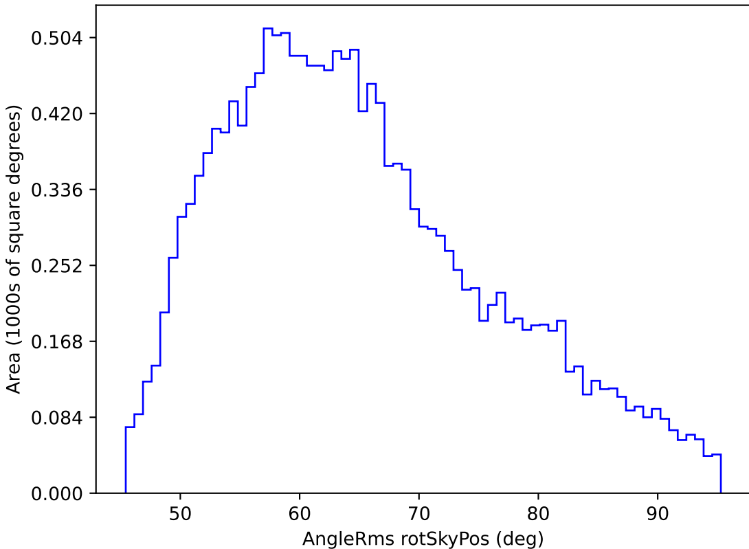
no_high_blob_v3.3_10yrs WFD y band: AngleRms rotSkyPos
