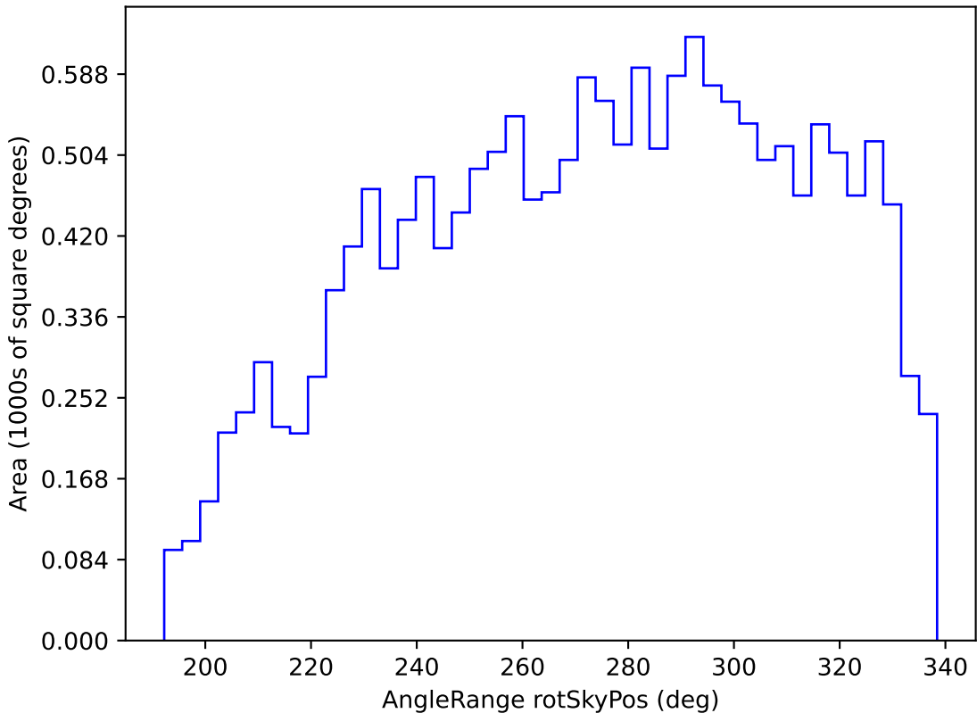
no_high_blob_v3.3_10yrs WFD y band: AngleRange rotSkyPos
